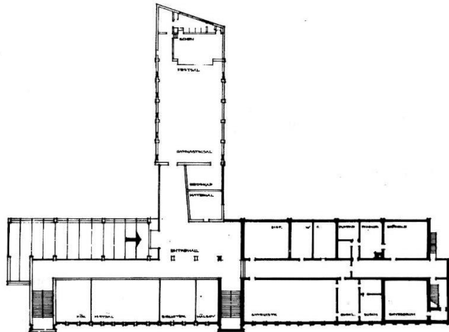
ENTRÉPLAN
